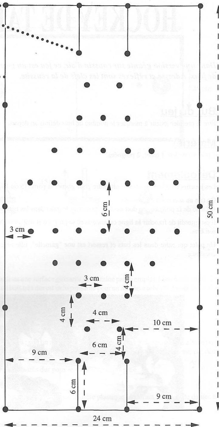
Plan du Billard Balinais
